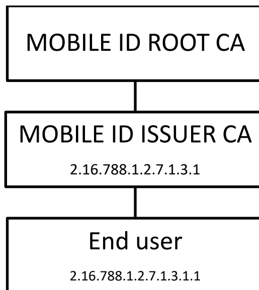
Fig-1: Mobile ID PKI CAs Hierarchy
